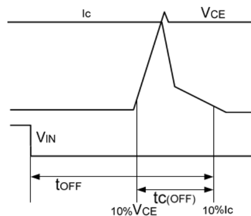
(b) 关断
